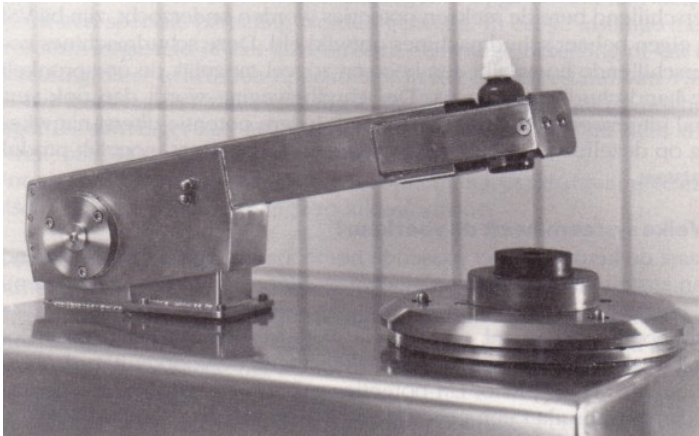
Figuur 2: 10-100 ml verticale schudmachine. Het flesje wordt in een houder met perslucht vastgeklemd en maakt 100 schudslagen tegen een verzwaard rubberen blok.
