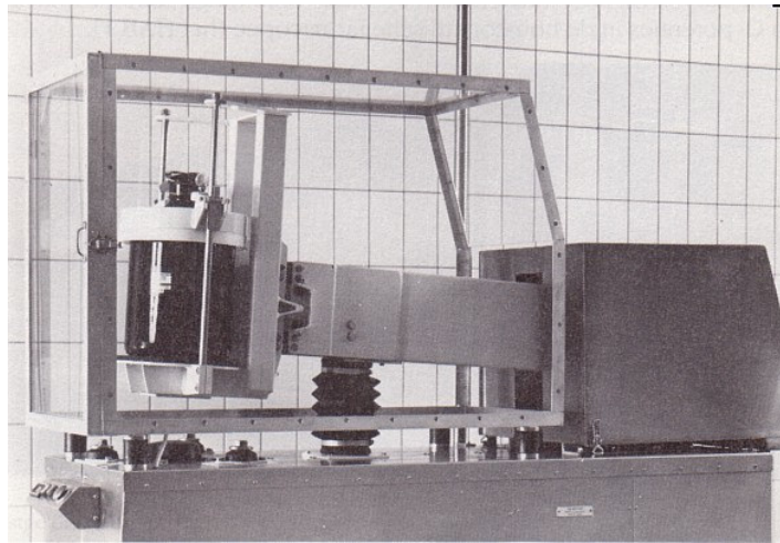
Figuur 1: 5 - 10 liter verticale schudmachine, maakt exact 100 slagen per potentieerstap. Fles met houder wordt tegen een 300 kg zwaar, van rubber voorzien, contragewicht geschud.
